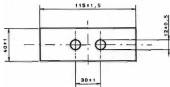
Teil Nr.10.20 Decklasche 2xM10
