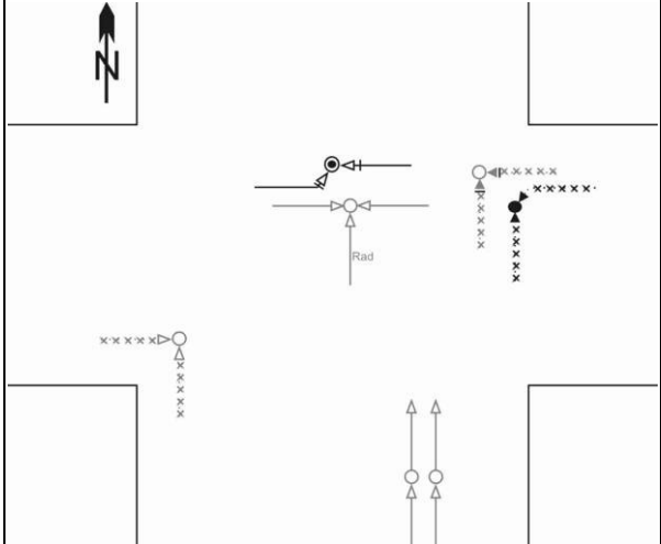
Unfalldiagramm 3-Jk(SP) bzw. (P) 2002 – 2004:
